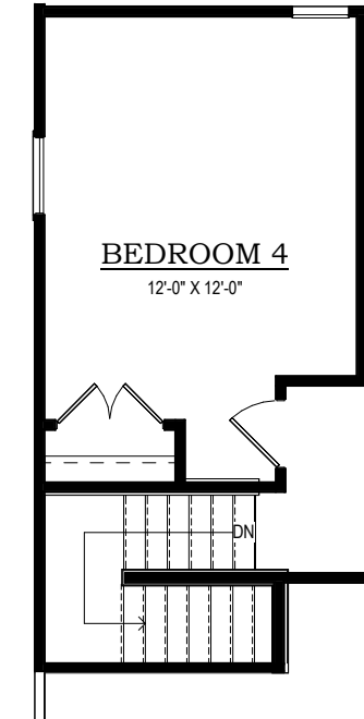
4TH BEDROOM IN LIEU OF LOFT Option #15122
